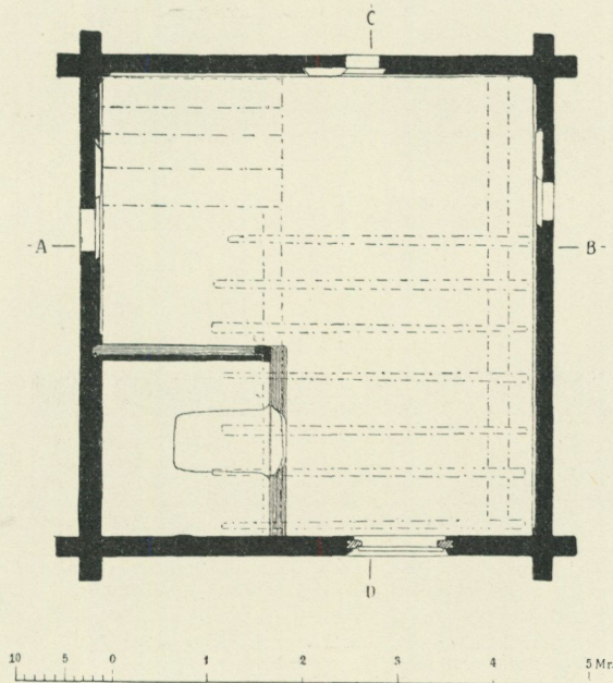
33. Plan af rökstugbadstugan från Rörkullen.
