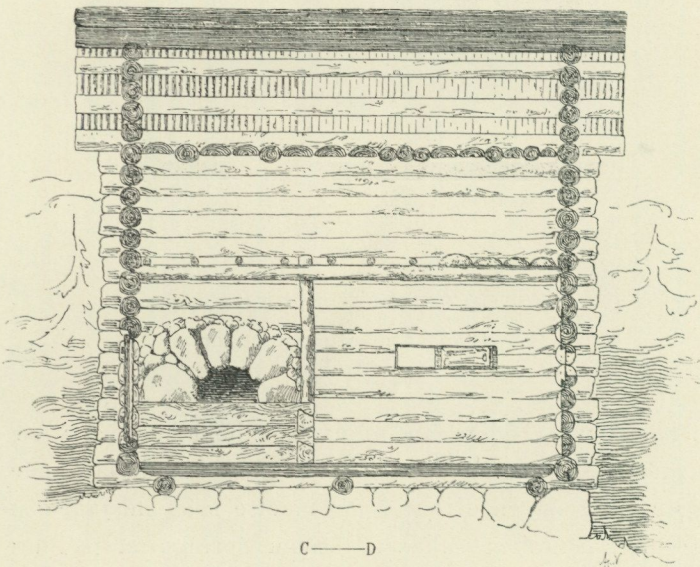
34, 35. Rökstugbadstugan från Rörkullen. Tvär- och längdsnitt.
