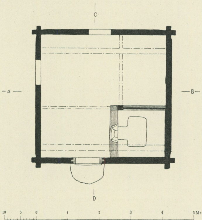
38. Plan af pörtet Damstugan.
