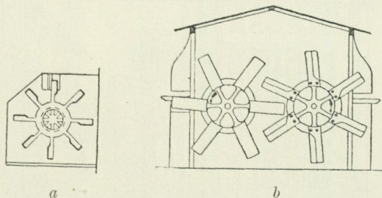
Fig. 14 a, b . Skäkthjul. Ur Lexikon der gesammten Technik und ihrer Hilfswissenschaften, herausgegeben v. Otto Lueger, Art. Flachsspinnerei.
