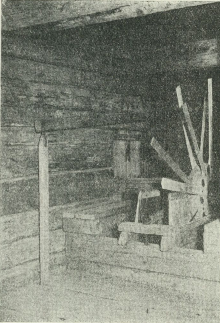
Fig. 11. Visar tydligare skaffötterna jämte de delar (ett tvärträ och en järnskrav) som hålla dessa i fixt läge. Längs väggen, ungefär mitt emellan golv och tak, sträcker sig »pådraget», d. v. s. den hävstång varmed stämbo-sluckan (jfr fig. 2) kan höjas och sänkas. Från änden av pådraget löper en annan stång ned genom golvet. Med den regleras stämbolet, då man befinner sig i underhuset.
