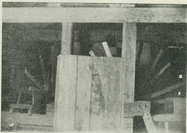
Fig. 9. Övra våningen med de båda skäkthjulen. Vid det högra hjulet ett bås av bräder, avsett att hindra skäv och avfall från att slungas omkring på golvet. Båset utmynnar nedåt i en avfallsränna, synlig i fig. 5.
