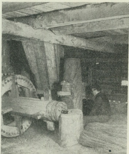
Fig. 5. Interiör från underhuset. T. v. kronstocken med kronhjulet. Tätt bortom kronhjulet synes trillen. T. h. hammaren, som lyftes av de på kronstocken synliga armarna. I fonden en avfallsränna ledande ned från övra våningen. I taket bjälkar och »bärås».
